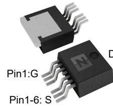
TO-263-6
